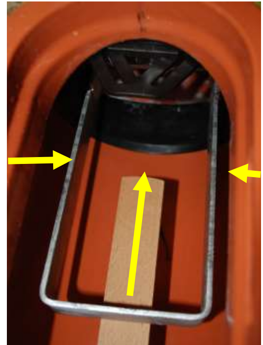
Montageholz hochkant einlegen, Ausbauspanne zusammendrücken und durch Innenteil durchschieben
